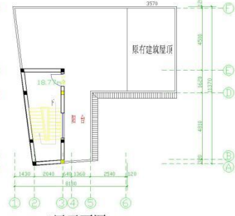
三层平面图 1:100
