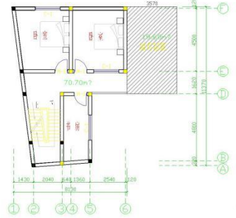
二层平面图 1:100
