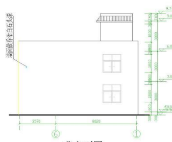
背立面图 1:100
