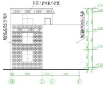
右侧立面图 1:100
