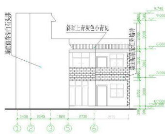
正立面图 1:100
