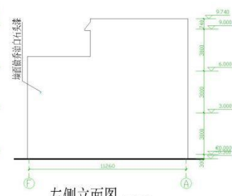
左侧立面图 1:100
