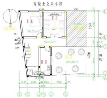
一层平面图 1:100
