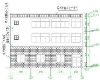
正立面图 1:100
