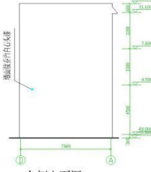
左侧立面图 1:100
