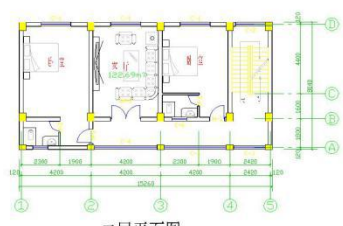
二层平面图 1:100
