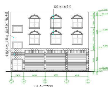
背立面图 1:100
