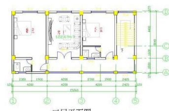
三层平面图 1:100
