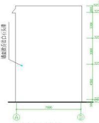
右侧立面图 1:100
