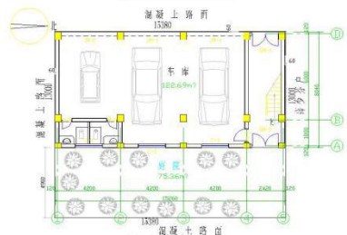
一层平面图 1:100
