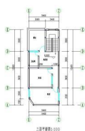
三层平面图 1:100
