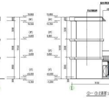
③-③ 剖面图 1:100
