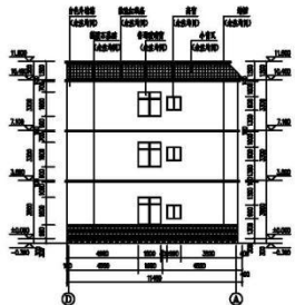
C-C剖面图 1:100
