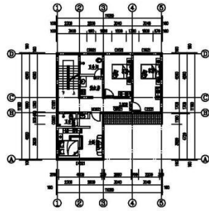
三层平面图 1:100 本层建筑面积: 94.57平方米
