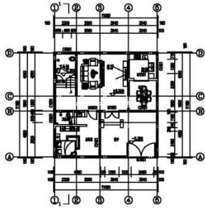
二层平面图 1:100 本层建筑面积: 94.57平方米 总建筑面积: 283.71平方米
