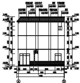
D-D剖面图 1:100
