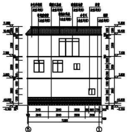
B-B剖面图 1:100
