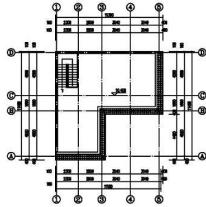
地下室平面图 1:100
