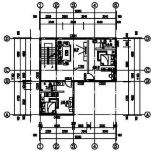
四层平面图 1:100 本层建筑面积: 94.57平方米
