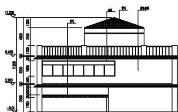
①-①立面
