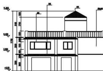
②-②立面
