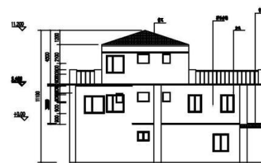
③-③立面
