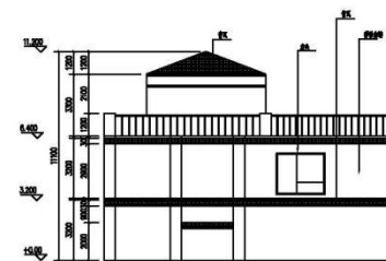
④-④立面
