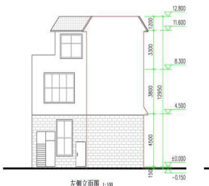
左侧立面图 1:100
