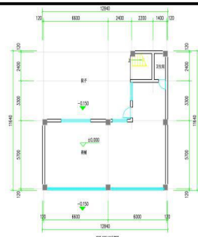
一层平面图 1:100
