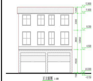
正立面图 1:100
