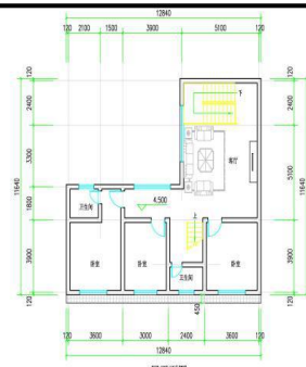
二层平面图 1:100
