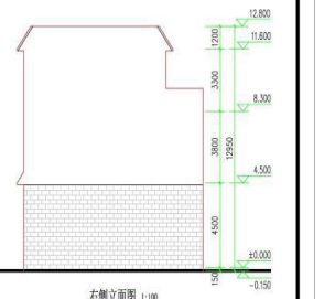
右侧立面图 1:100
