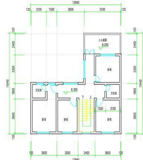
三层平面图 1:100
