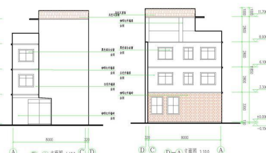
D-A 立面图 1:100
