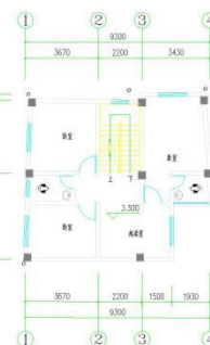
二层平面图 1:100 71.44平方米
