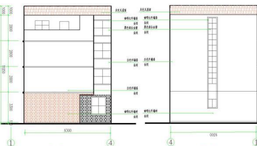
1-4 立面图 1:100
