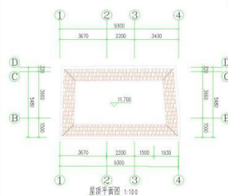
屋顶平面图 1:100
