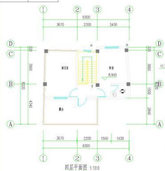
四层平面图 1:100 56.23平方米
