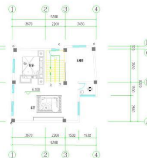
三层平面图 1:100 71.44平方米
