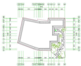
总平面图 1:100
