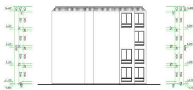
正立面 1:100
