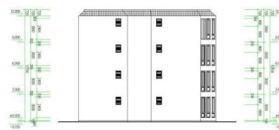
侧立面 1:100
