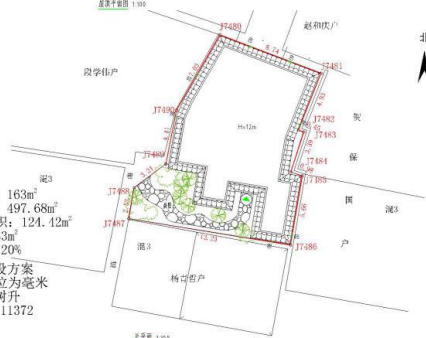
总平面图 1:100
