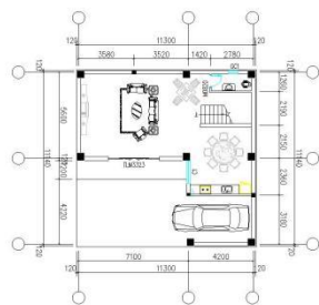
一层平面图 1:300 建筑面积: 96.23 m²
