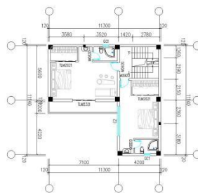
二层平面图 1:300 建筑面积: 96.23 m²
