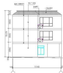
C~A立面图 1:300
