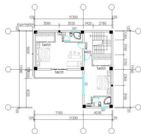
三层平面图 1:300 建筑面积: 96.23 m²
