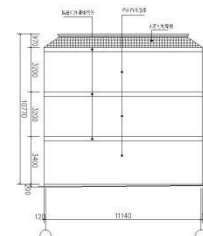
A~C立面图 1:300
