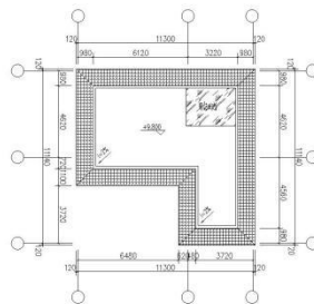
屋面平面图 1:300
