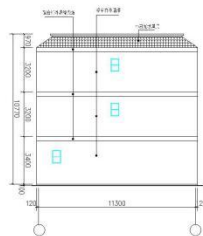
③~①立面图 1:300
