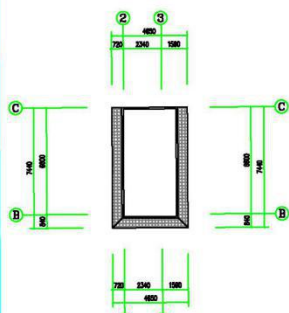
层平面图 1:100
