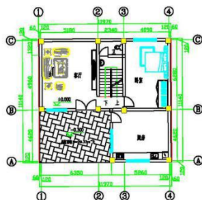
一层平面图 1:100 本层建筑面积: 102.68m 2 总建筑面积: 336.61m 2 一层建筑占地面积: 102.68m 2
