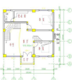
二层平面图 1:100
