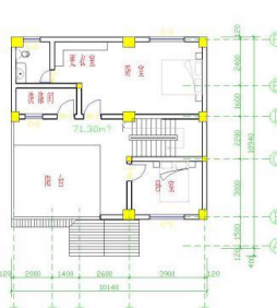
三层平面图 1:100
