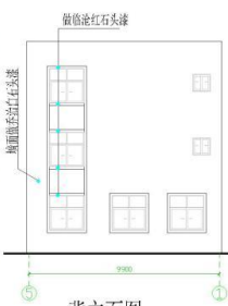
背立面图 1:100
