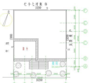
屋顶投影总平面图 1:100
