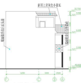
左侧立面图 1:100
