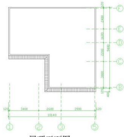
屋顶平面图 1:100
