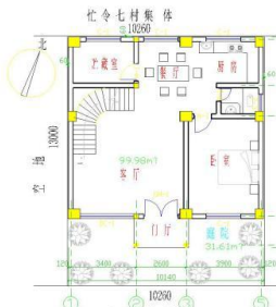
一层平面图 1:100
