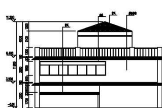
①-①立面
