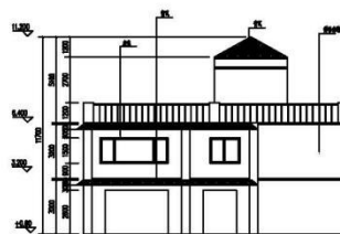
②-②立面
