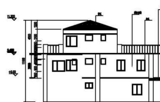
③-③立面
