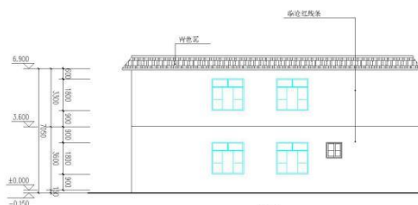
正立面图 1:100
