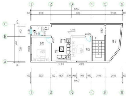
二层平面图 1:100 本层建筑面积: 91.64
