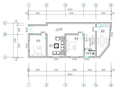
一层平面图 1:100 本层建筑面积: 108.01 总建筑面积: 199.65 平方米
