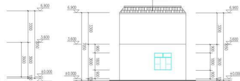
右立面图 1:100
