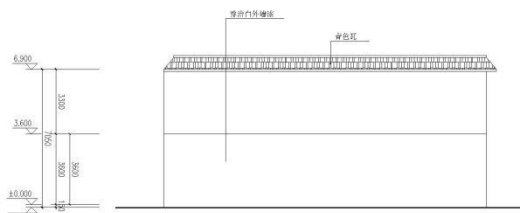
背立面图 1:100
