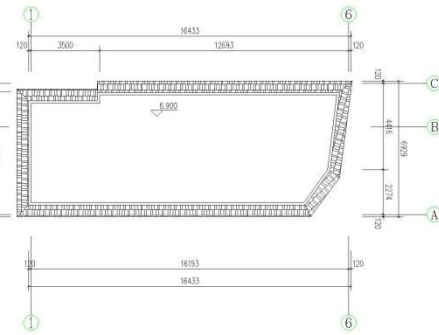
屋顶平面图 1:100
