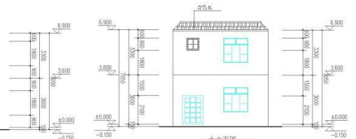
左立面图 1:100
