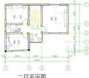
二层平面图 1:100
