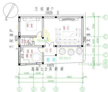
一层平面图 1:100
