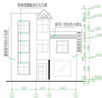
正立面图 1:100
