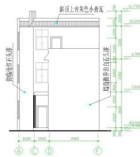
右侧立面图 1:100
