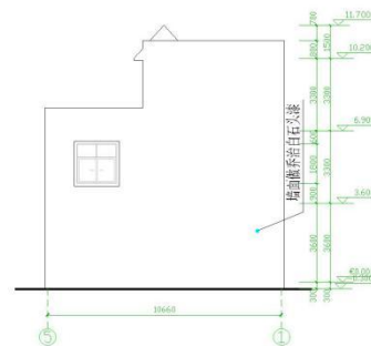
背立面图 1:100
