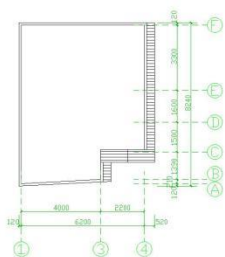
屋顶平面图 1:100
