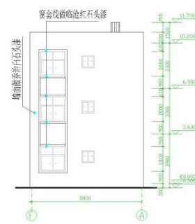
左侧立面图 1:100
