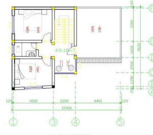
三层平面图 1:100
