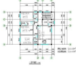
二层平面图 1:100
