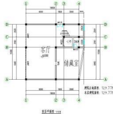
一层平面图 1:100
