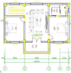
二层平面图
