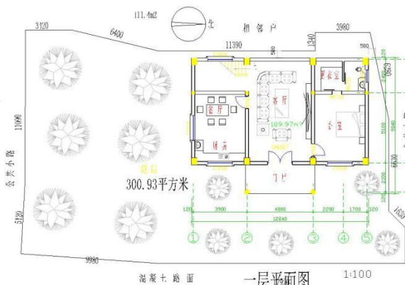
一层平面图
