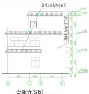
右侧立面图 1:100
