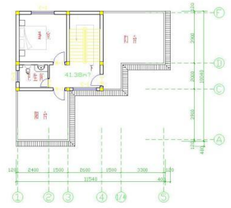
三层平面图 1:100
