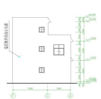
左侧立面图 1:100
