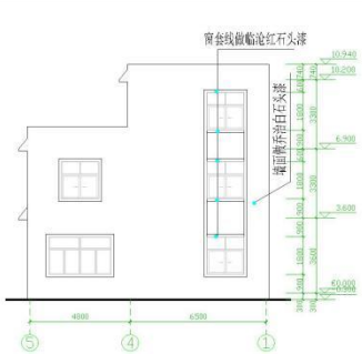
背立面图 1:100
