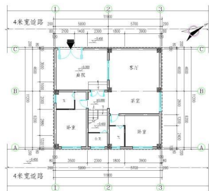
总平面图 1:100
