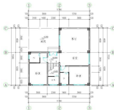
三层平面图 1:100
