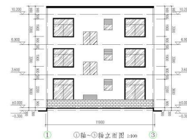
③轴~⑤轴立面图 1:100
