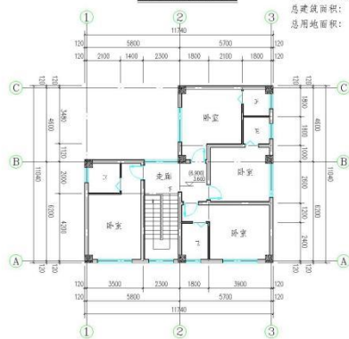
一层平面图 1:100
