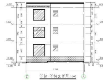
④轴~⑥轴立面图 1:100
