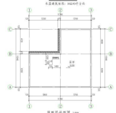
屋面平面图 1:100
