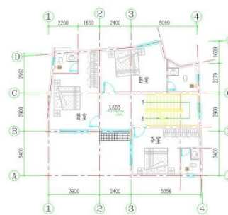
二层平面图 1:100
