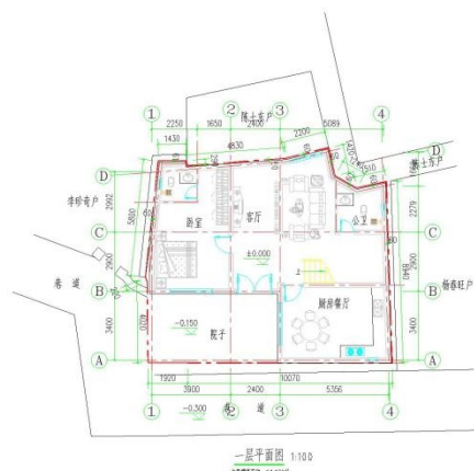
一层平面图 1:100
