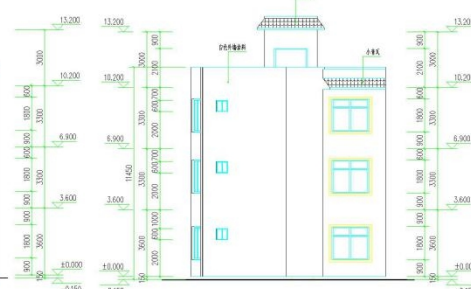
左側立面图 1:100
