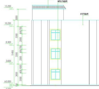
背立面图 1:100
