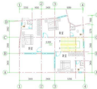
三层平面图 1:100
