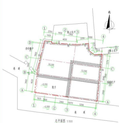
总平面图 1:100
