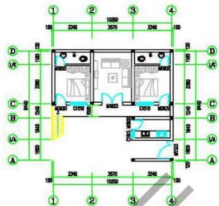
一层平面图 1:250
