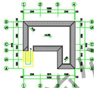
屋面平面图 1:250
