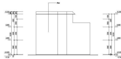
⑥-①轴立面图 1:100
