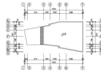
屋顶平面图 1:100
