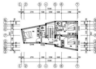
二层平面图 1:100 本层建筑面积70.03m 2
