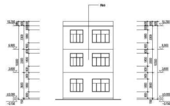
①-⑥轴立面图 1:100
