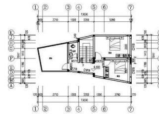
三层平面图 1:100 本层建筑面积54.55m 2
