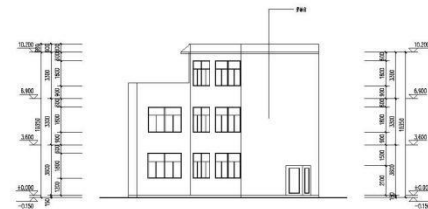
①-⑥轴立面图 1:100
