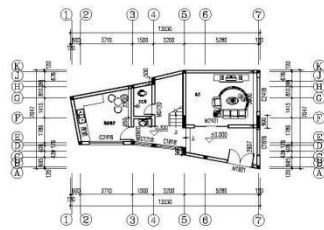
一层平面图 1:100 本层建筑面积70.03m 2 总建筑面积194.61m 2
