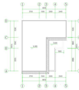
屋顶平面 1:100
