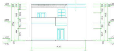
④-④轴立面图 1:100
