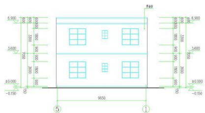
③-③轴立面图 1:100
