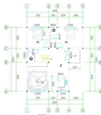
一层平面 1:100 本层建筑面积: 96.06 平方米 总建筑面积: 175.12 平方米
