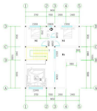
二层平面 1:100 本层建筑面积: 79.06 平方米
