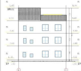
前立面图
