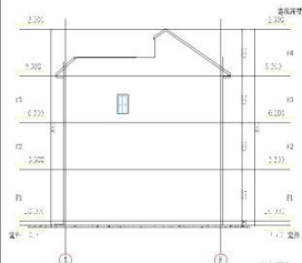
正立面图
