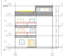
后立面图
