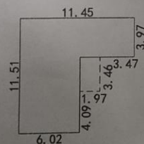
1层平面图
