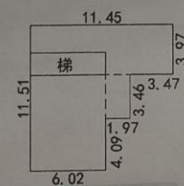
2层平面图
