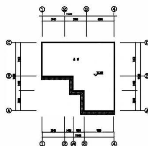
屋顶平面图 1:100
