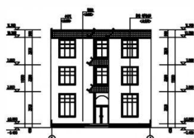
①-④ 立面 1:100
