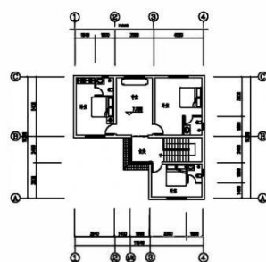
三层平面图 1:100
