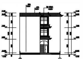
②-③ 立面 1:100
