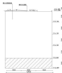
左侧面图
