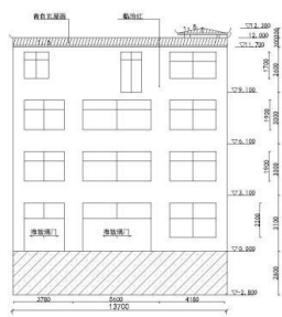
正立面图
