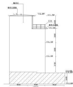
右侧面图
