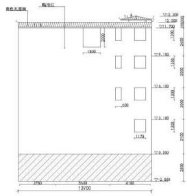
背立面图
