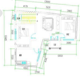
新建一层平面图 1:100
