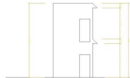
左侧立面图 1:100
