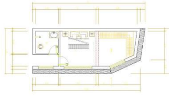
二楼平面图 1:100
