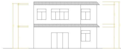
正立面图 1:100
