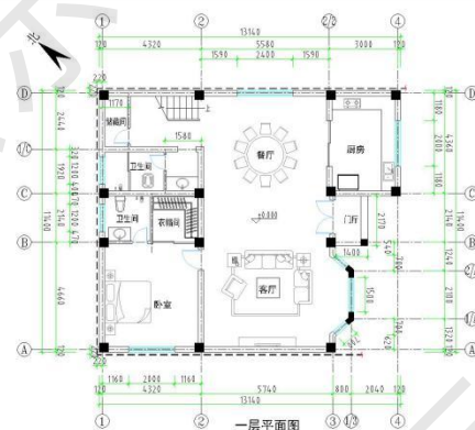
一层平面图
