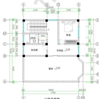
三层平面图
