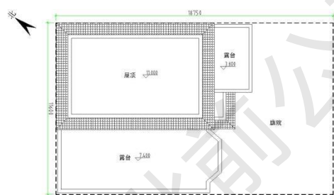
屋顶投影总平面图
