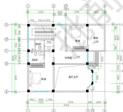
二层平面图
