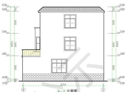
4-1 立面图
