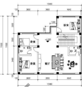
二层平面布置图 1:100 二层建筑面积：120.13m²
