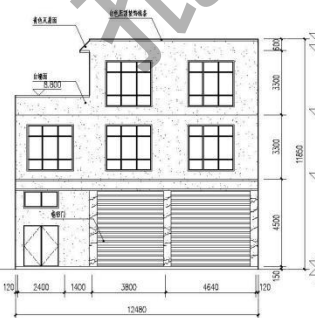
建筑东立面图 1:100
