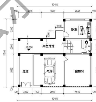
一层平面布置图 1:100 一层建筑面积：99.44m² 一层建筑占地面积：120.13m² 本栋建筑总面积：284.5m²
