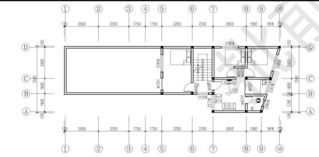
二层平面图 1:100
