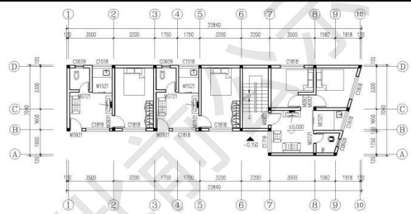
一层平面图 1:100
