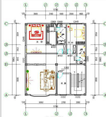
三层平面图 1:100 本层建筑面积为: 170.40平方米 总建筑面积为: 611.28平方米
