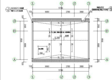
屋顶平面布置图 1:100
