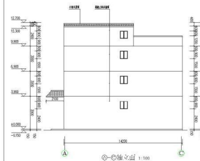
①-②轴立面 1:100
