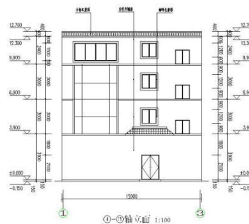
①-③轴立面 1:100
