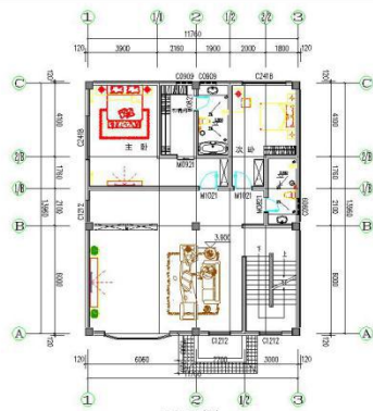
二层平面图 1:100 本层建筑面积为: 170.40平方米 总建筑面积为: 611.28平方米
