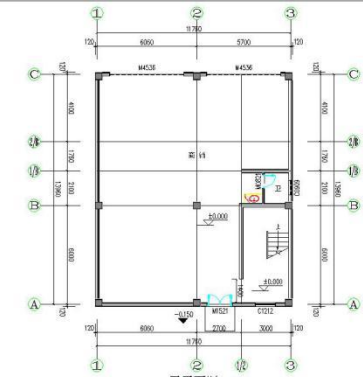
一层平面图 1:100 本层建筑面积为: 170.40平方米 总建筑面积为: 611.28平方米
