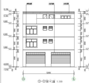
③-①轴立面 1:100
