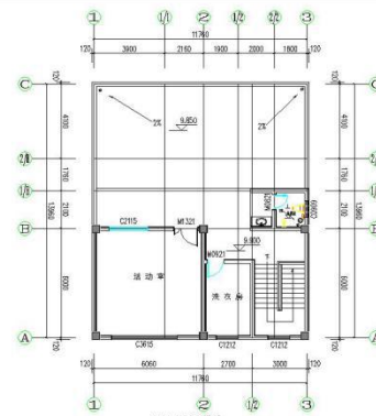
四层平面图 1:100 本层建筑面积为: 170.40平方米 总建筑面积为: 611.28平方米
