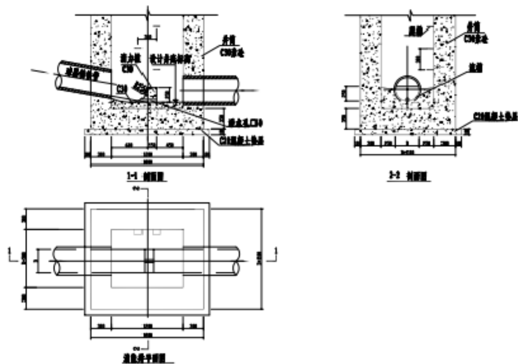
消能井大样图
