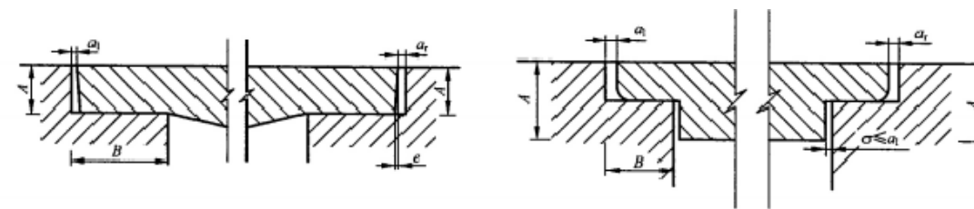
检查井盖结构形式图
