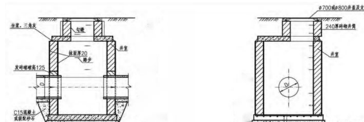
混凝土沉泥井大样图
