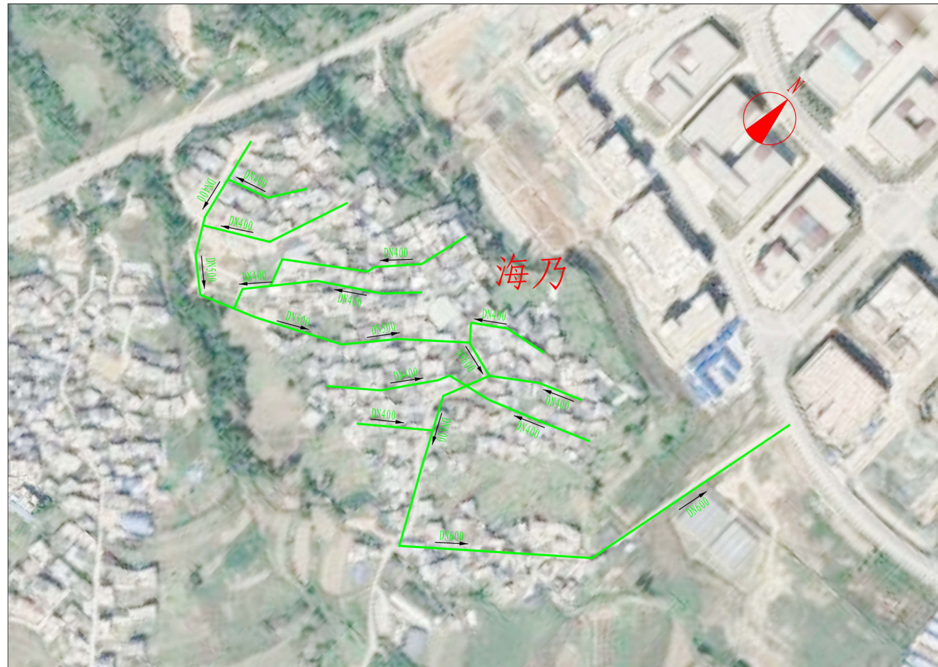
海乃片区排水防涝治理示意图
