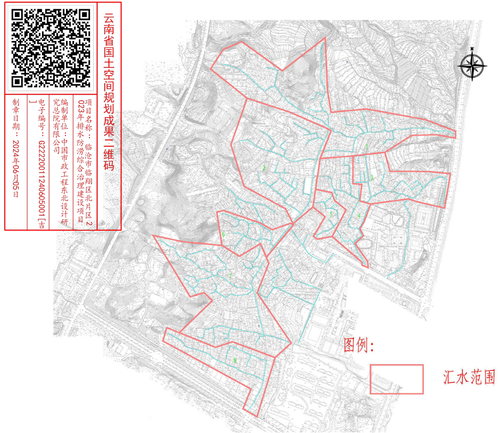
青华村片区排水防涝治理汇水范围图
