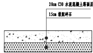
混凝土路面恢复大样图
