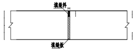
胀缝构造
