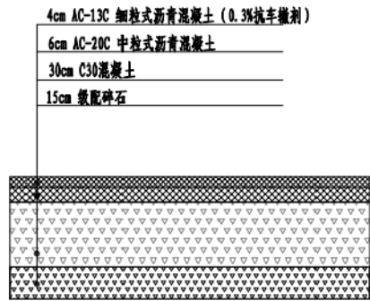
沥青路面恢复大样图
