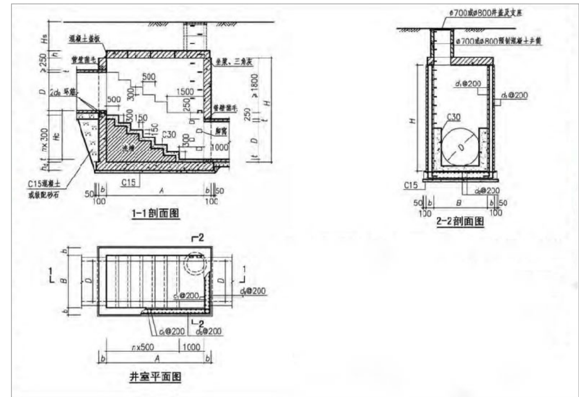
阶梯式混凝土跌水井大样图
