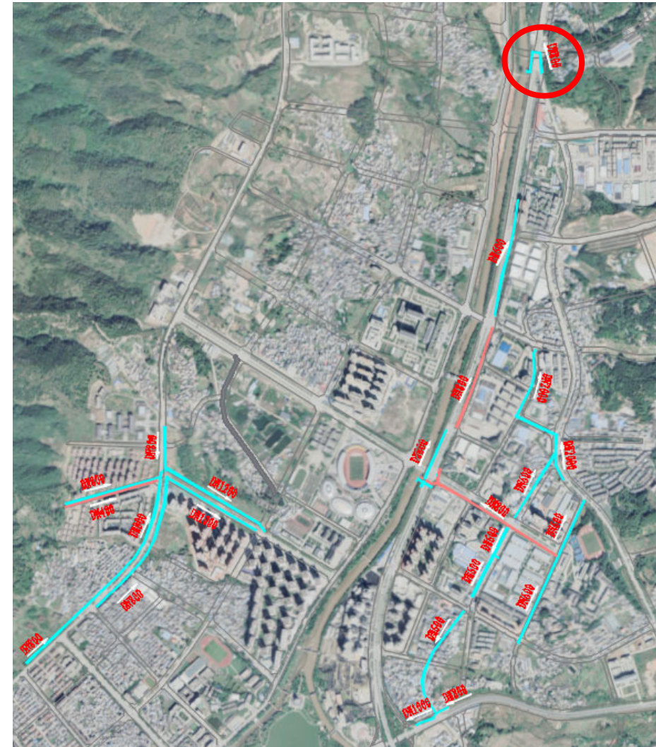
恒春大道与缅宁大道交叉口治理范围示意图
