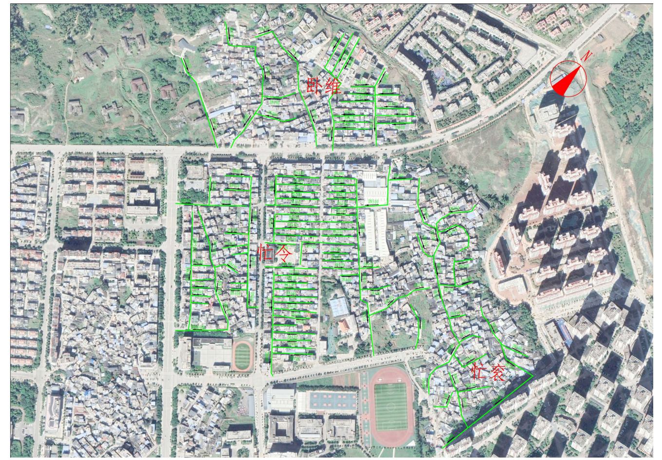
卧维、忙令、忙袞片区排水防涝治理示意图
